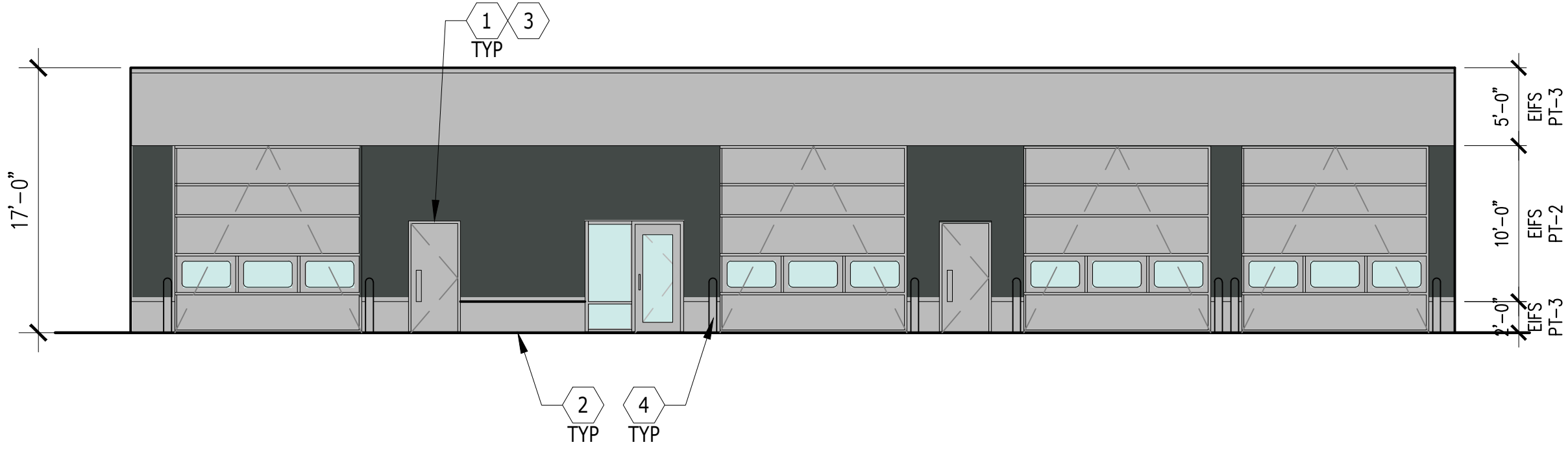
RIGHT ELEVATION SCALE: 1/8" 1
