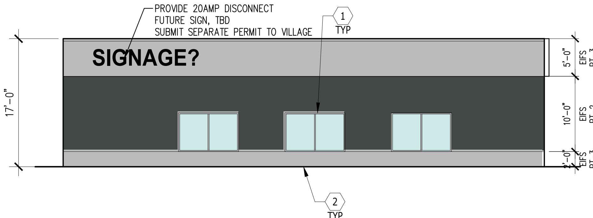
LEFT ELEVATION SCALE: 1/8" 3
