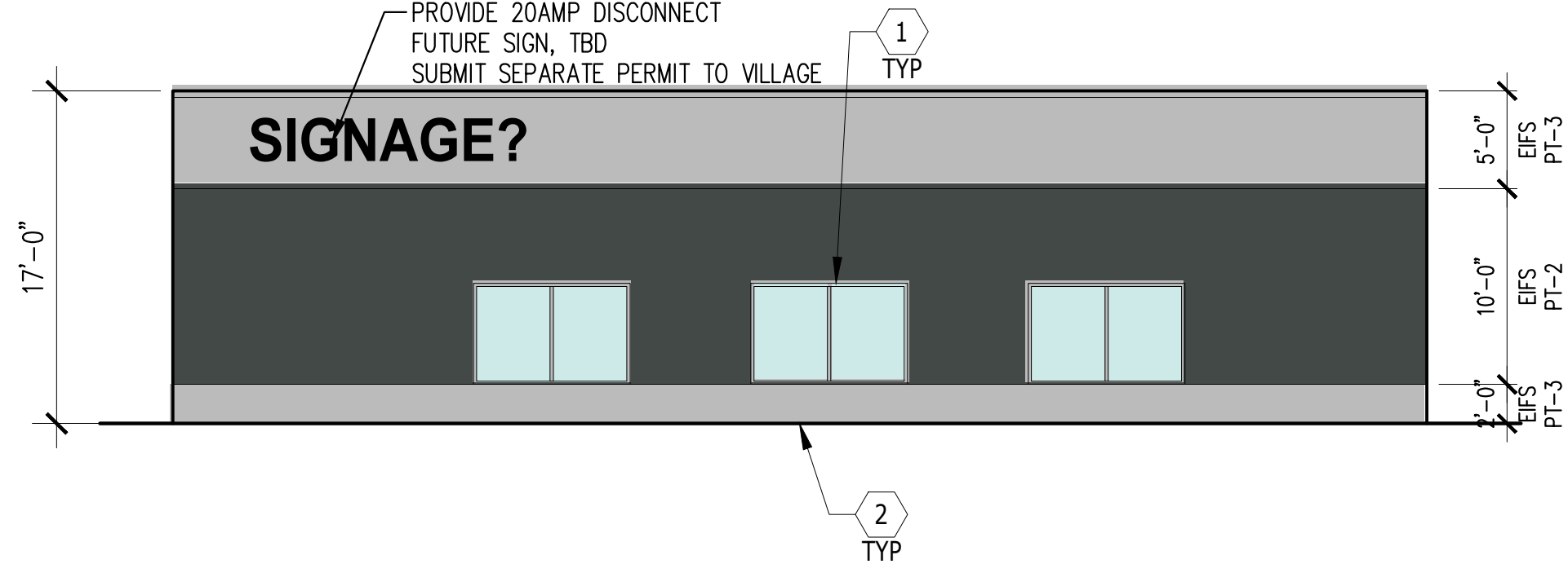
FRONT ELEVATION SCALE: 1/8" 2
