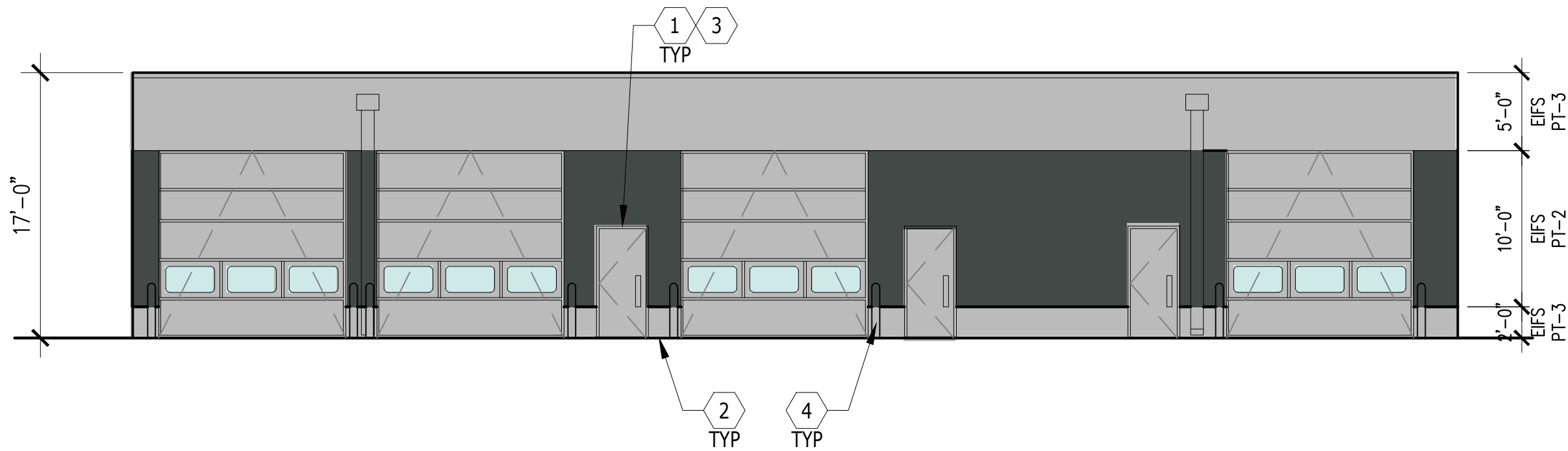
LEFT ELEVATION SCALE: 1/8" 4
